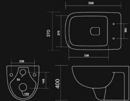
Size : 370 x 560 x 400mm 16 KG
